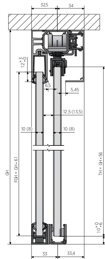
Querschnitt-Zeichnung Festglas-Set mit Glas Komplett-Set
